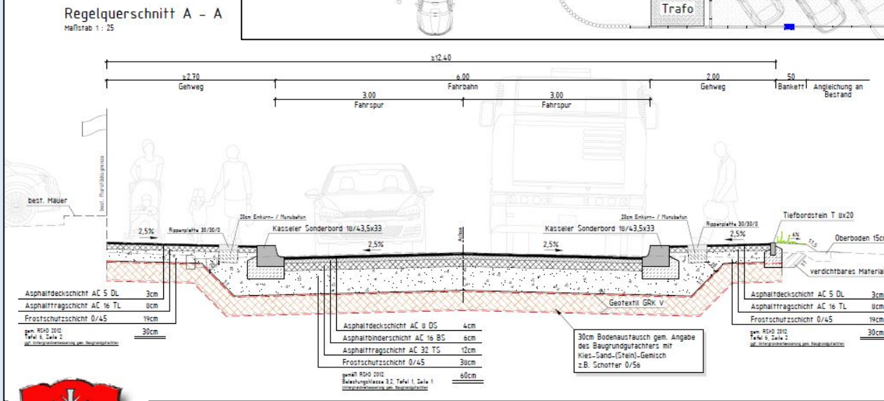
Querschnitt
