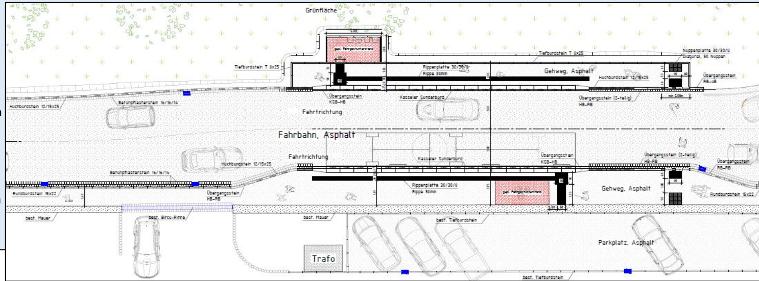
Lageplan
