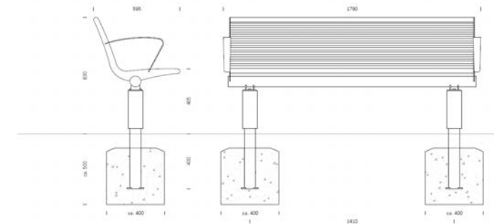
BODENVERANKERUNG ZUM EINBETONIEREN, EINBAUTIEFE 400 MM
